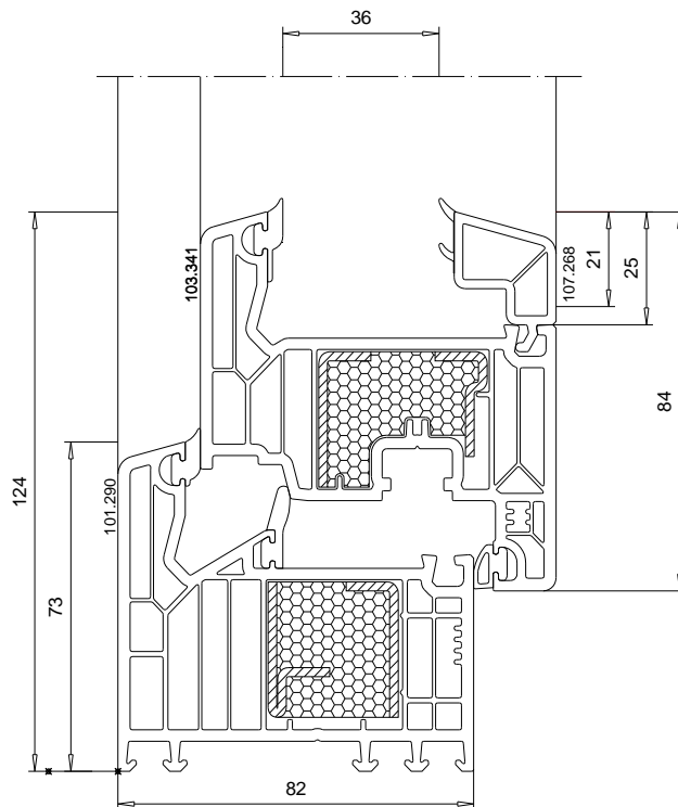
Bild 1 Darstellung des Querschnitts
