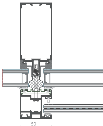
Mocowanie balustrady do słupa fasadowego
