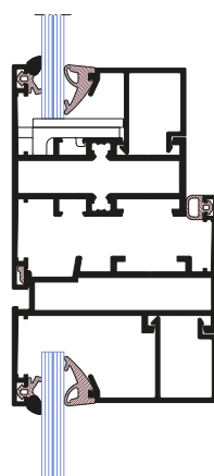
Okno podawcze – przekrój pionowy
